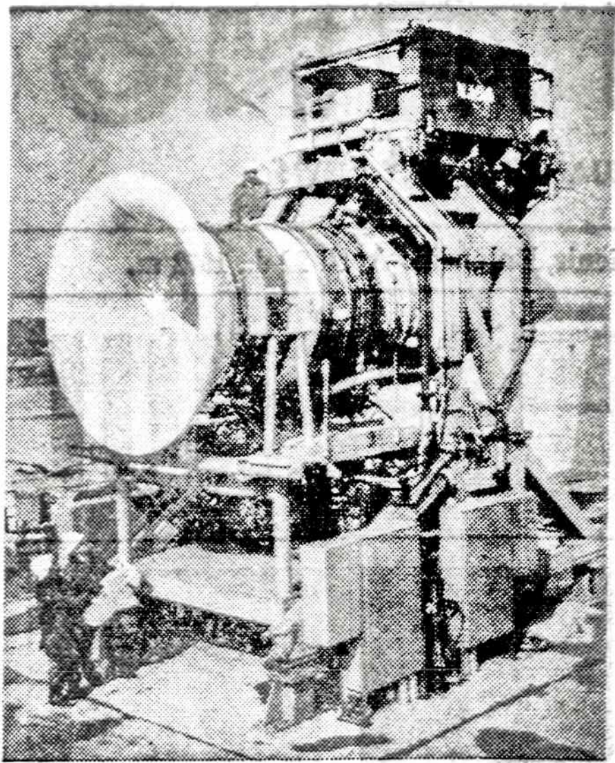
NASA Lewis Bandymų centre prie Clevelando inžinieriai išbando naują sprausminį motorą, kuris pasižymi savo "tylumu". Atelityje daug keleivinių lėktuvų bus aprūpinti "tyliais motorais".
