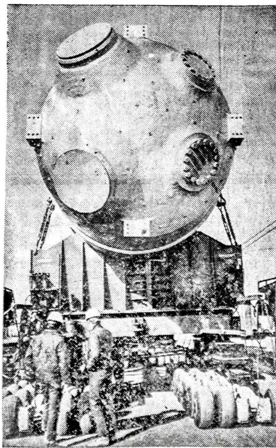
Naujas elektros jėgainės generatorius 65 mylias keliavo 5 dienas. Tas 375 tonų milžinas buvo gabenamas specialioje 145 pėdų ilgumo platformoje su 128 ratais. Generatorius skirtas naujai branduolinių jėgainių Mineral, Virginijoje.
