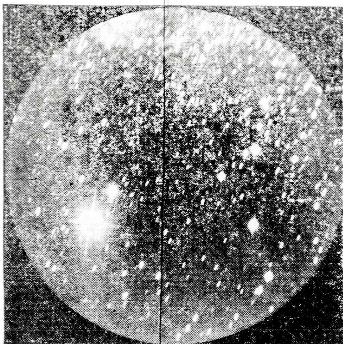
Apollo 16 astronautas John Young skridamas erdvėje nufotografavo daug dangaus ir žemės vaizdų. Čia matoma Paukščių Tako nuotrauka. Didelis kūnas kairėje, apačioje, yra Jupiterio planeta.
