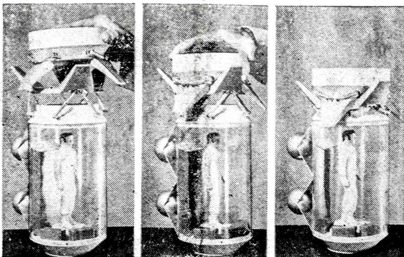
Amerikoje suprojektuotas "Docking Module" — Amerikos ir Sovietų Sąjungos erdvėlaivų prisijungimo stoties modelis. Viršutinė jos dalis pritaikyta sovietų laivo susijungimo mechanizmui priimti, o apatinė dalis tinkama susijungti su JAV Apollo laivu. Amerikiečiai ir sovietų astronautai galės šios stoties pagalba pareiti iš vieno erdvėlaivio į kitą.
