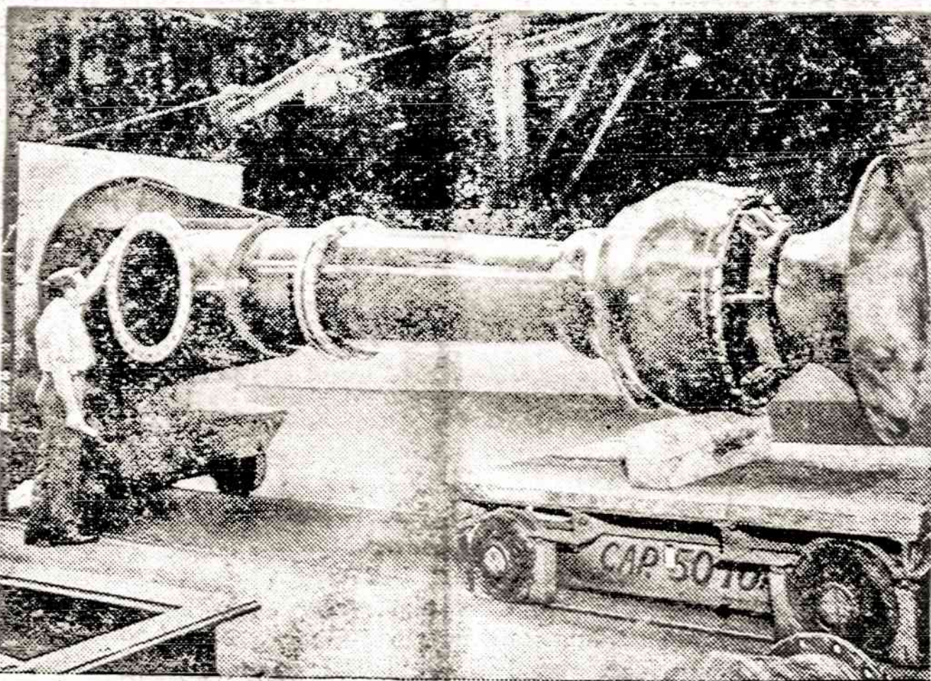
Ne milžiniška žvakidė ar pučiamasis instrumentas, bet vandens pompas dalis, kuri bus siunčia-ma į Trinidadą, žibelo valyklai. Pompa pagamino Allis - Chalmers bendrovė.
