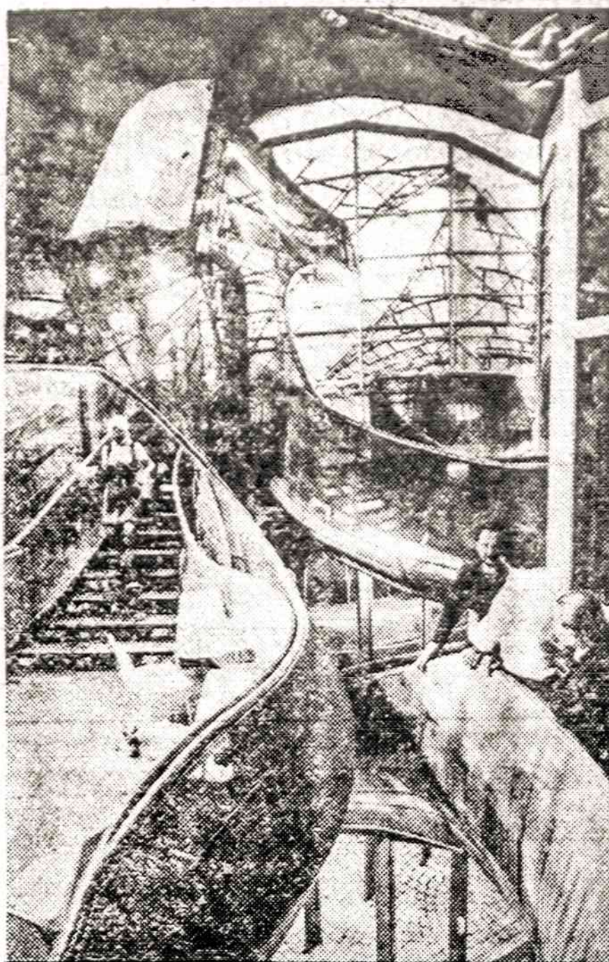
V. Vokietijos inžinieriai ir architektai statydami Muencheno Olimpiadai pastatus, panaudojo daug naujovių. Nuotraukoje matosi plaukymo salės vingiuoti laiptai.
