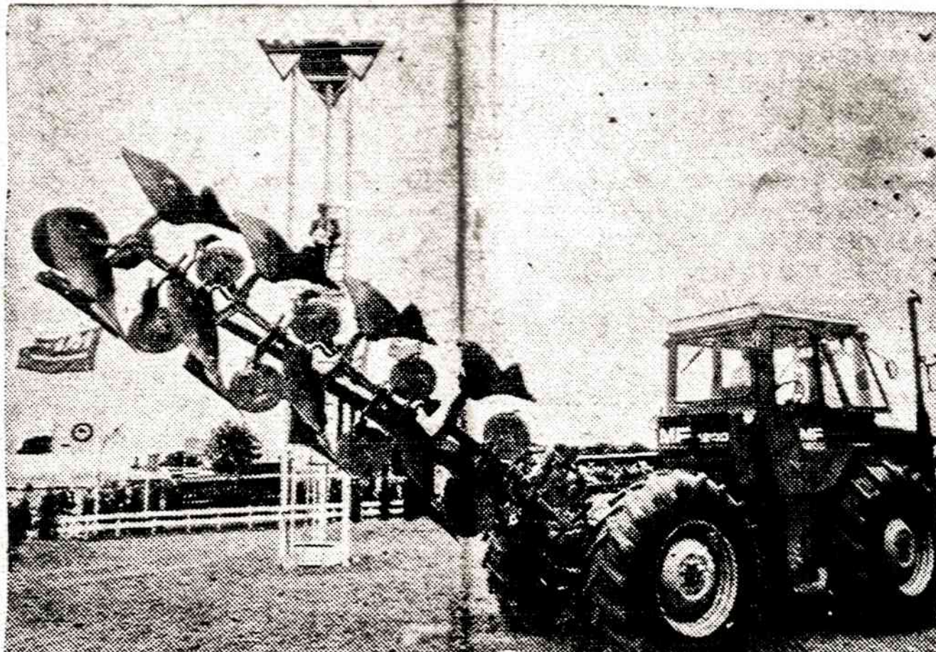
Civilizuotas traktorius, parodytas Anglijos žemės ūkio parodoje. Kabina yra vėsinama, turi minkštą sėdynę ir klimą. Traktorius kelia mažai triukšmo ir virpėjimą sumažina guminiai blokelai.
