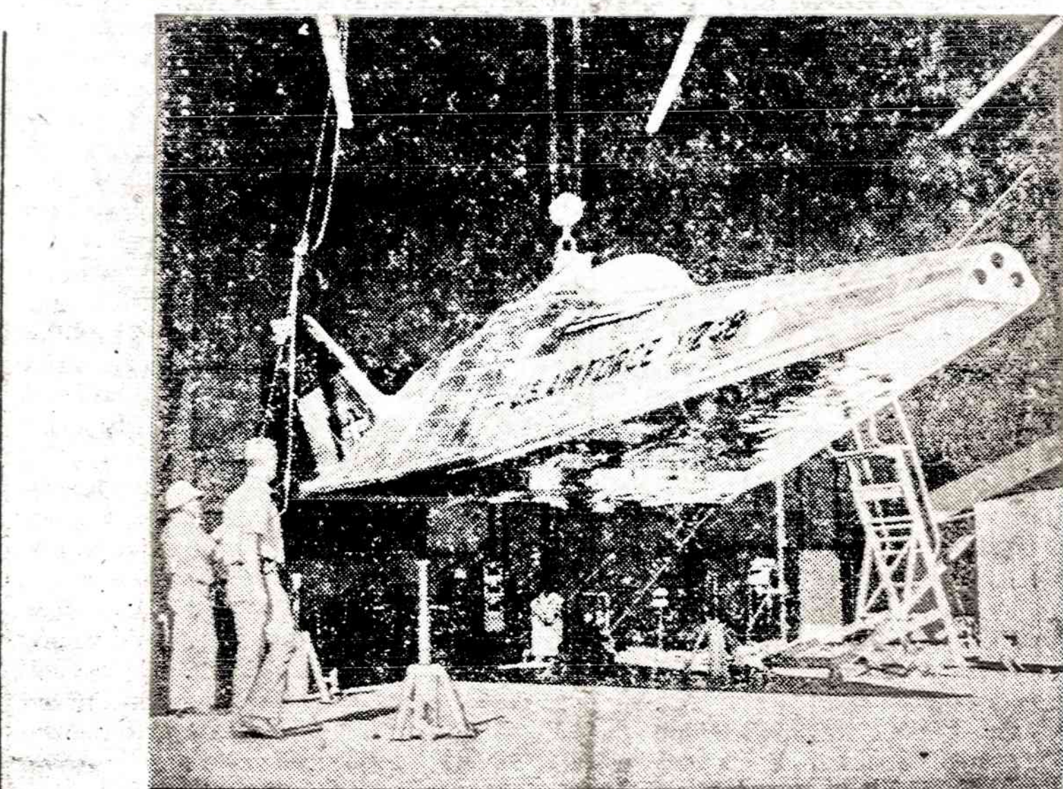
Specialių uždavinių lėktuvai, naudojami tyrinėjimams, vadinami "Lifting Body". Juos paprastai iškelia didieji B-52 bombonešiai, o toliau jie pa'ys skrenda raketinio motoro pagalba. Šis LF lėktuvas X-24-B yra pats naujasis. Jis čia nuleidžiamas ant žemės Edwards aviacijos bazės angare.
