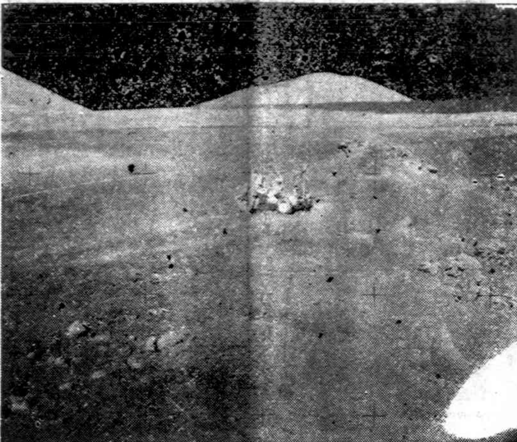
Mėnulio vaizdas. Tolyje matosi LR (Lunar Rover) su astronautu Schmitt. Fotografavo astronautas Eugene Cernan.
