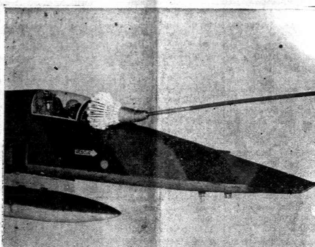
Nepagalvokime, kad nuo lėktuvo kas valo dulkes. Tai vamzdis, kuriuo Kanados CF-5 lėktuvas pripilamas skysto kuro iš skraidančio tanko-lėktuvo.
