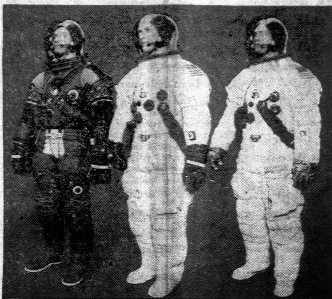
Astronautų drabužių mados greit nesikeičia, bet jau yra kostiumai, kurie naudojami skirtingiems uždaviniams. Kairėje spaudimo rūbų kompleksas, viduryje — šiluminis micrometeoroidų kostiumas su erdvėlaivio viduje dėvimam pirštinei. Dešinėje — drabužiai nešiojami išėjus iš laivo erdvėje.
