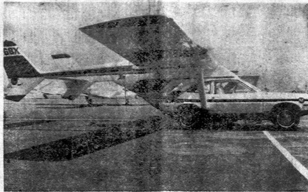
Nauja transporto priemonė "AVE Mizar". Priekyje, vietoj lėktuvo nosies įtaisytas Fordo "Pinto" automobilis. Lėktuvo sparnai ir uodega prie automobilio pritaisoma per dvi minutes. Tiek pat trunka automobilį atkabinti. Visa kombinacija gali skraidyti ore ar važinėti žeme. Dar nebaigti šios mašinos bandymai. Lėktuvą varo spraguminis Cessna Skymaster motoras, įtaisytas už pakelįje sparnu.
