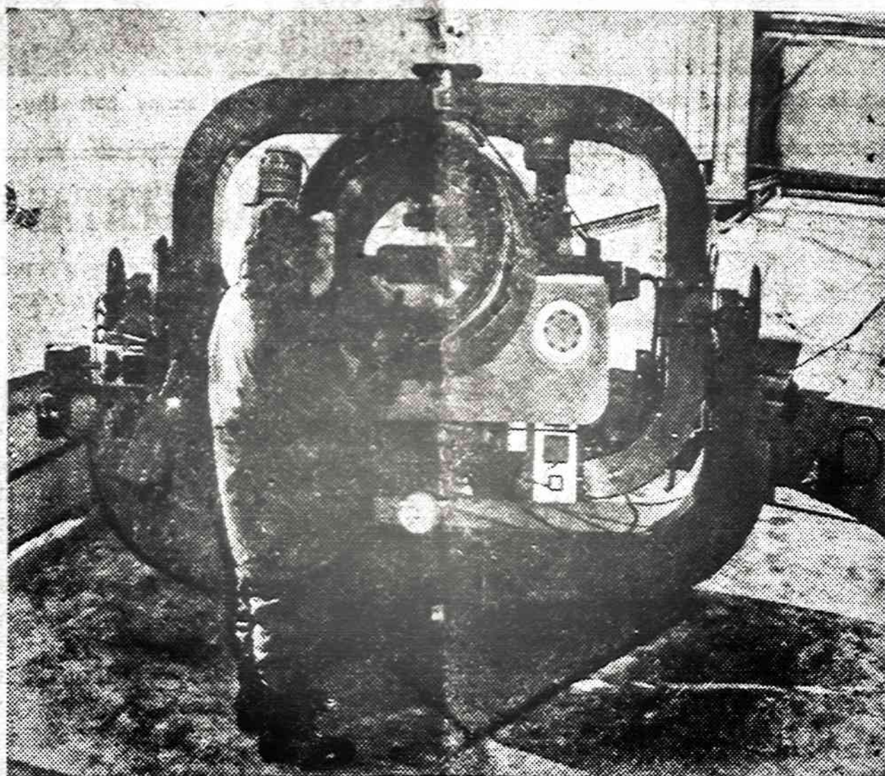
Labai tikslus žemės satelitų sekimo aparatas — Baker - Nunn kamera, kuri gali nufotografuoti sviedinio didumo šviesos tašką 25,000 mylių atstume. Aparatas yra naudojamas šiaurės Amerikos Oro Gynybos komandos bazėje, Cold Lake Aliaskoje.
