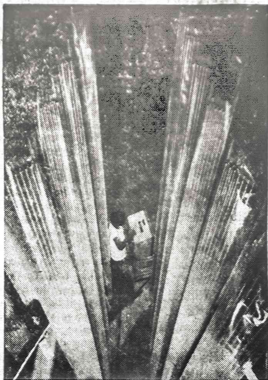
Wilmington, N. C. gaminami metalo virbalai, kurie sujungti į pluoštus, naudojami branduolinių energijos gamybai komerciniuose reaktoriuose.
