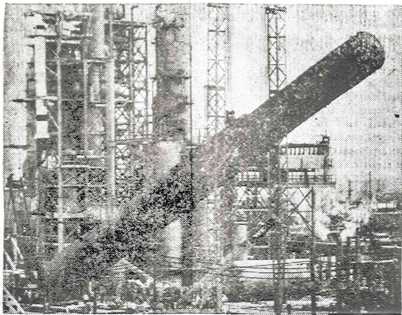
Texas City, Texas, naujai statoma Marathon Oil bendrovės rafinerija. Jos 600 tonų sunkumo bokštas, pakeliamas į am skirtą vietą, atrodo, kaip patrankos vamzdis.
