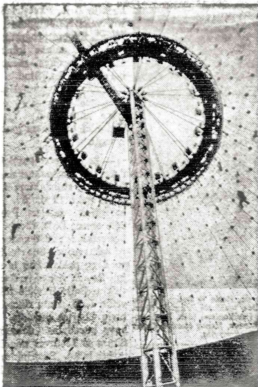
Amerikos paviljonas Expo-74, Spokane, Wash., atrodo lyg didelio voro nuostatus tinklas. Ant plieninių lynų buvo užtiestas plonas plastmasinis uždangalas.
