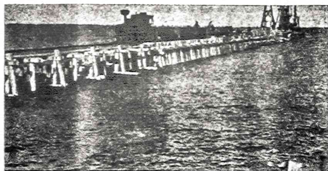
Šventosios uostas 1939 m. Statomoji krantinė.
