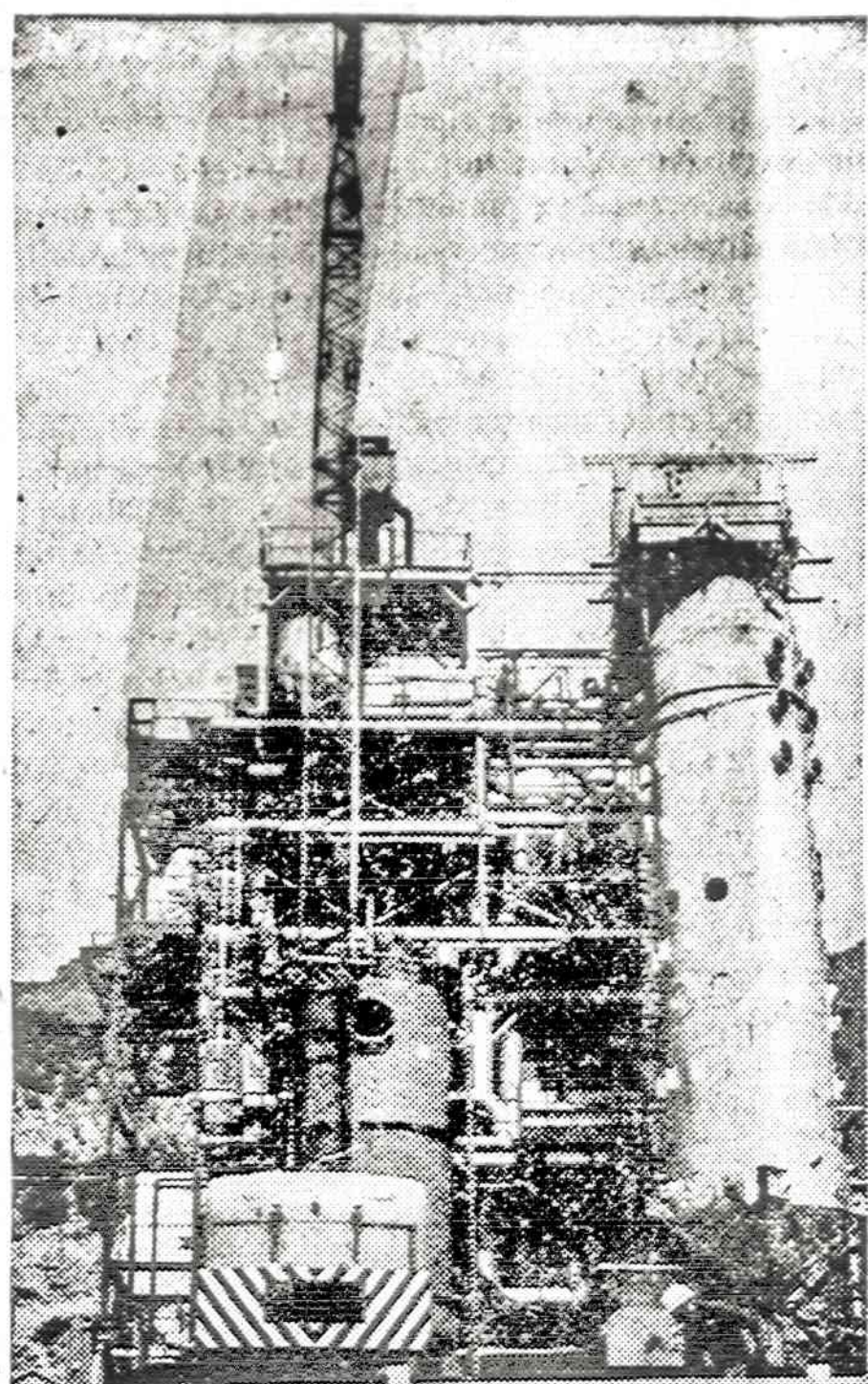
Paraho bendrovė Anvil Points, Colo., sutrina naftos pilną uolieną į dulkes ir kaitinimo metodu iš jos išgauna naftą. Sakoma, kad vien tik Rocky Mountain srityje yra 700 milijonų statinių naftos, tik jos išėmimas iš uolų yra sudėtingas ir ilgas procesas.
