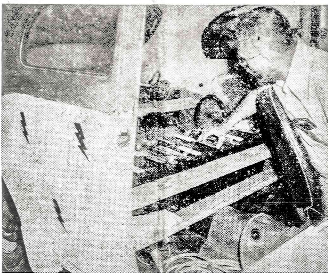
Bill Vernedeo, dirbas Marshall Erdvės Skridimų Centre, Alabamoje, išėmė iš savo Volkswageno automobilio užpakalinę sėdynę ir įtaisė toje vietoje 10 baterijų po 90 amperų kiekvieną. Jis turi įrengęs 27 arklio jėgų motorą, kuris pasiekia 50 mylių per val. greitį. Suvažinėjus 40 mylių, baterijas reikia iš naujo pakrauti.
