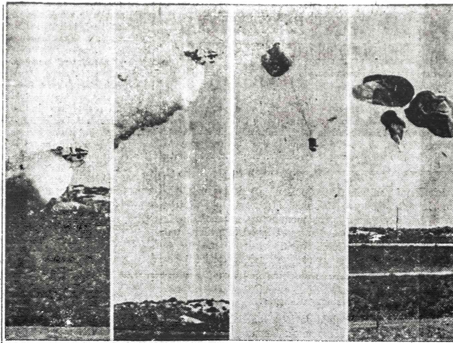
Rockwell International bendrovė išbando naujus lakūnų gelbėjimo metodus. Kairėje nuo B-1 strateginio bombonešio atsiskiria atskira kapsulė su lakūnais. Kapsulė pakyla 507 pėdas virš lėktuvo, naudodama dvi nedideles raketas. Atitinkamoje aukštumoje išsiskleidžia parašiutai ir lakūnai nuleidžiami ant žemės.
