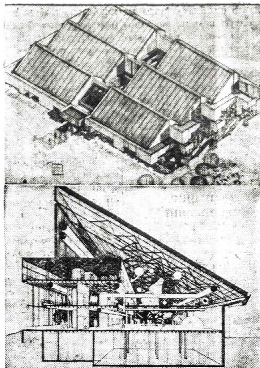
Owens-Corning Fiberglass Corp. kasmet skiria premijas už projektus, kaip išvystyti saulės spindulių energiją. Viršuje pirmą prizą laimėjęs Nevados universiteto projektas, kuriame pastato stogas turi 4,000 pėdų saulės spindulių rinkėją, kuris šildo pastatą. Apačioje panašus Virginijos Mokslo muziejaus projektas.
