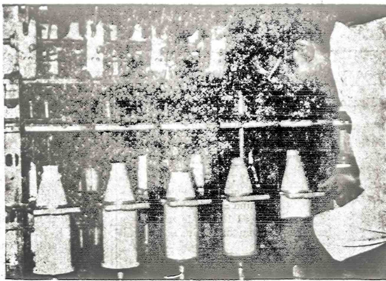
Pagrindinis žingsnis tapti audiniu: fibrinės pavijos automatiškai vyniojamos ant spūlių.
