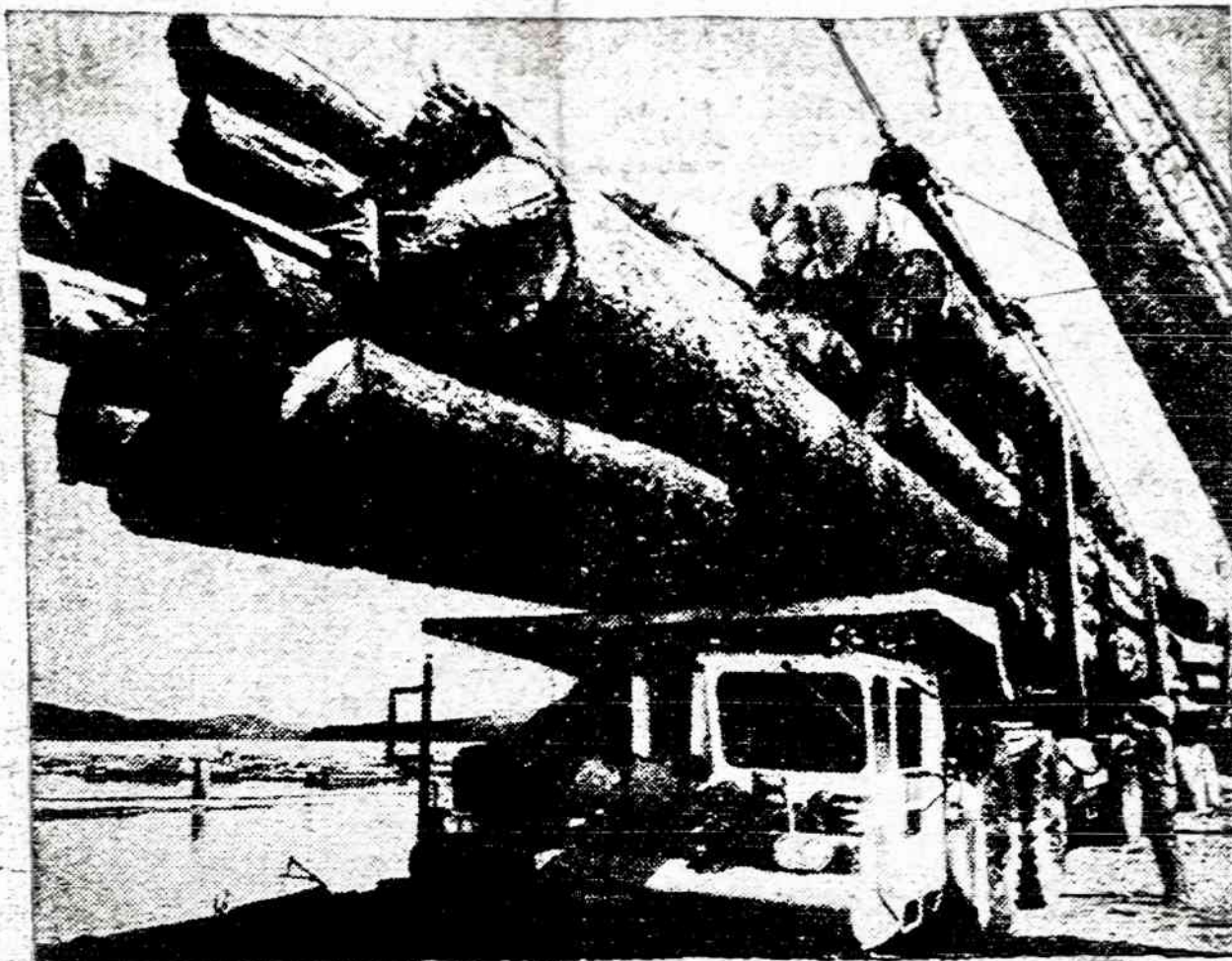
Kanadoje, britų Kolumbijoje, kanadiečiai pasigaminą naują sunkvežimį rastamą vežti. Padarytas specialus žemas dangtis, kad galėtų daugiau prikrauti ir vienu vežimu išvežti iš skynimų. Šitas stiprus keliaratis sunkvežimis vienu važiuoju gali išvežti 250 tonų rasti. Jeigu naujas sunkvežimis bus praktiškas, tai kanadiečiai daugiau jį pasistatys.
