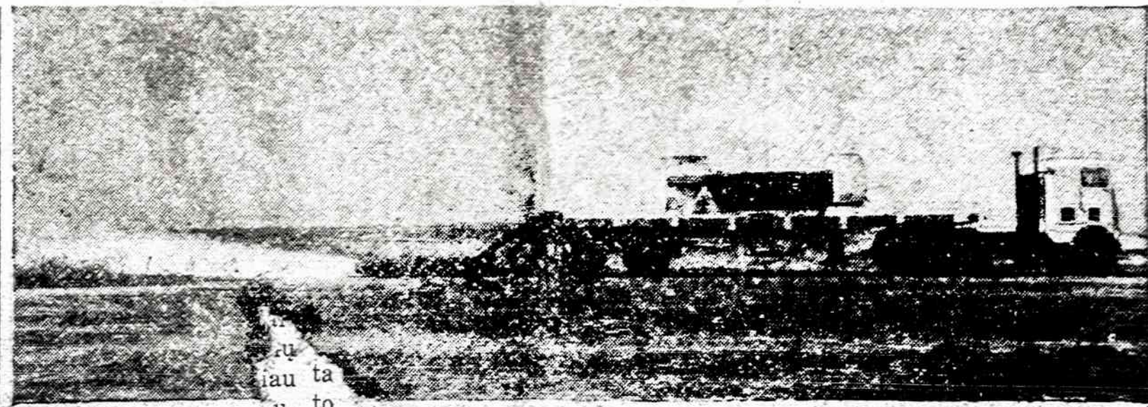
Iš tolo kontroliuojamas AS-14-00 reaktorius, važiuodamas 60 mylių greičiu, stuktelėjo į cementinę sieną. Smūgis buvęs toks stiprus, kad jis iššovė 22 tonas sveriantį atominės bombos luobą. Bandymus davo Sandia Laboratorijos specialistai Naujos Meksikos dykumose.
