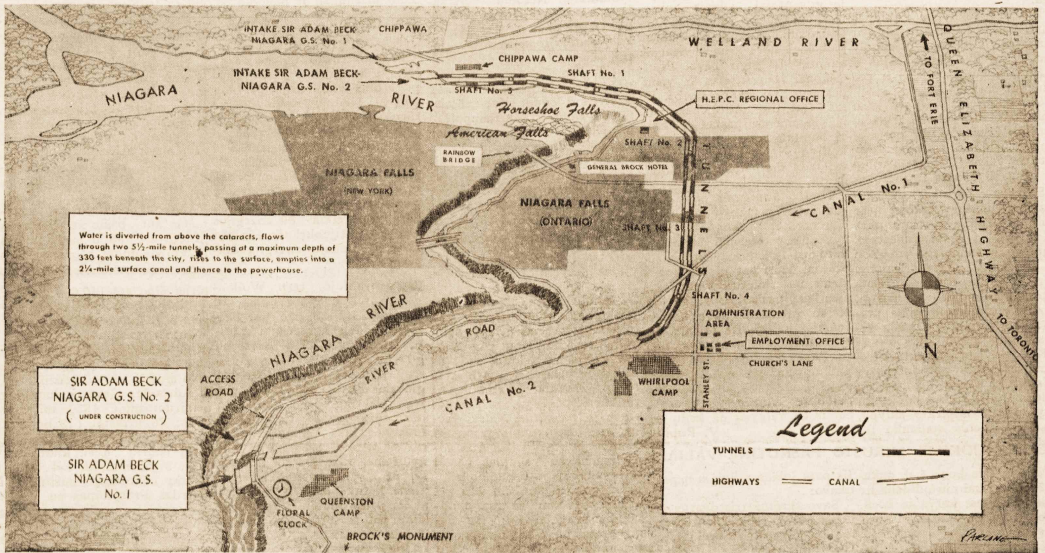
ONTARIO HYDRO'S NEW NIAGARA DEVELOPMENT — NIAGAROS UPĖS, KRIOKLIO, Miesto ir elektros jėgainių išvystymo planas. Jis parodo, kaip ir kur vedami tuneliai, kuriais bus nuleistas Niagaros vanduo, kuris bus įkinkytas į turbinas, kurios gamins elektrą.
