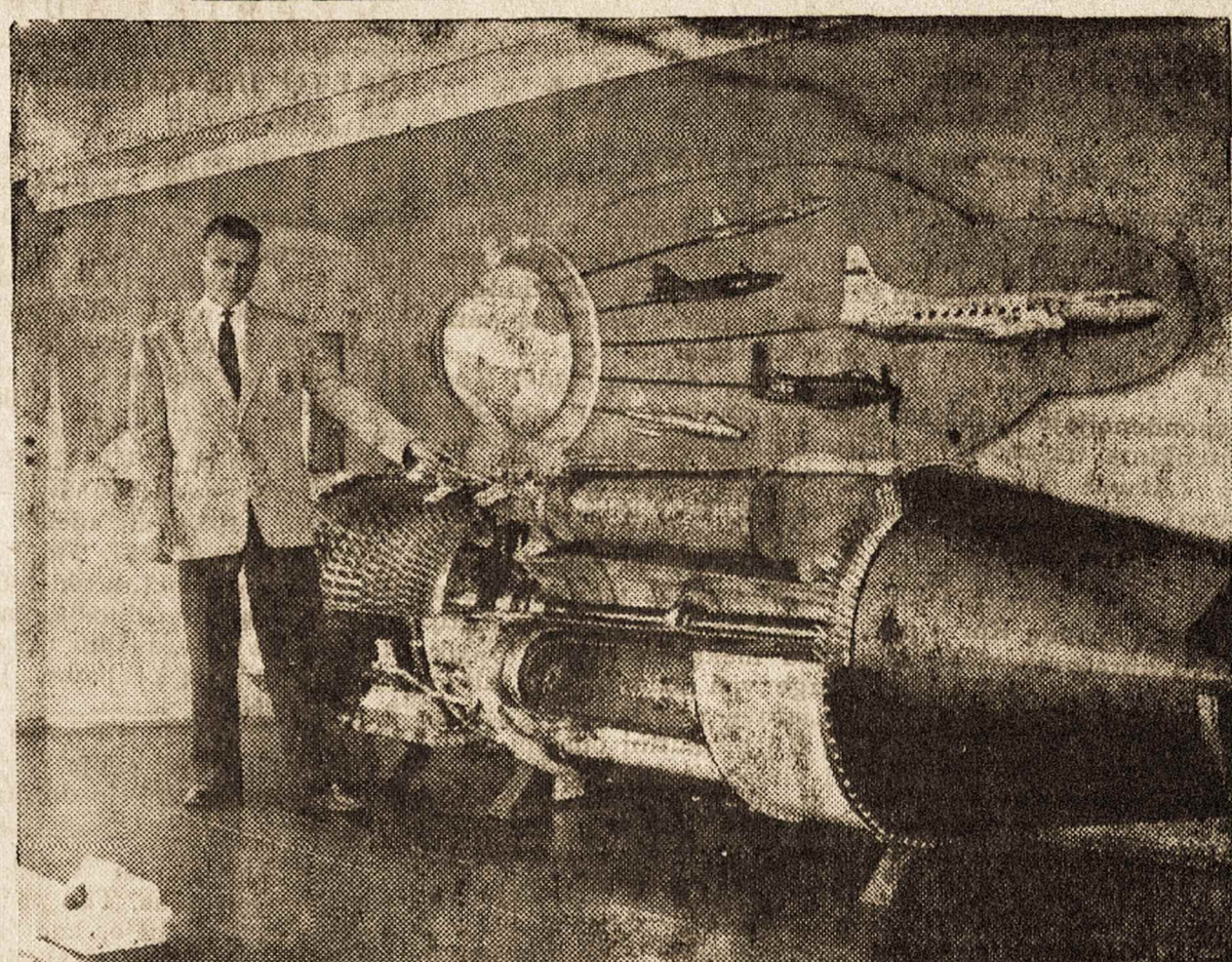
General Motors Bendrovės ruošiamame Progreso Parade bus parodytas didžiulis vei- kiantis permatomas sprausminis motoras, kartu bus paaikškinami sprausminio motoro veikimo principai. Progreso Paradas, keliaujanti mokslo paroda, susidedanti iš 24 eks- ponatų, kartu su 40 minučių vaidinimu scenoje, buvo įrengta prieš Kanados Nacionali- nės Parodos Princesės Vartus Toronte. Visa paroda yra nemokama ir buvo atidaryta publikai nuo liepos 19 iki liepos 23 d.
