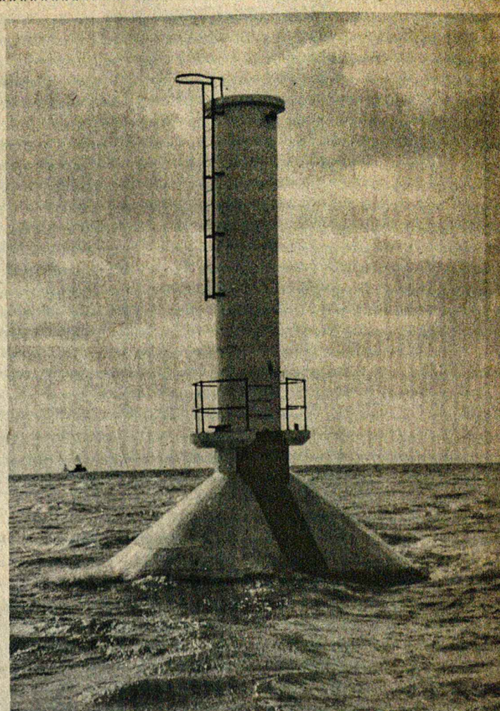
Svyturys Lake Erie ežere prie Detroit upės žiočių. Pastatė Department of Transport of Canada. Projektavo J.V. Danys (iš lietuvių inž. ir arch. suvažiavimo Ottawoje parodos).
