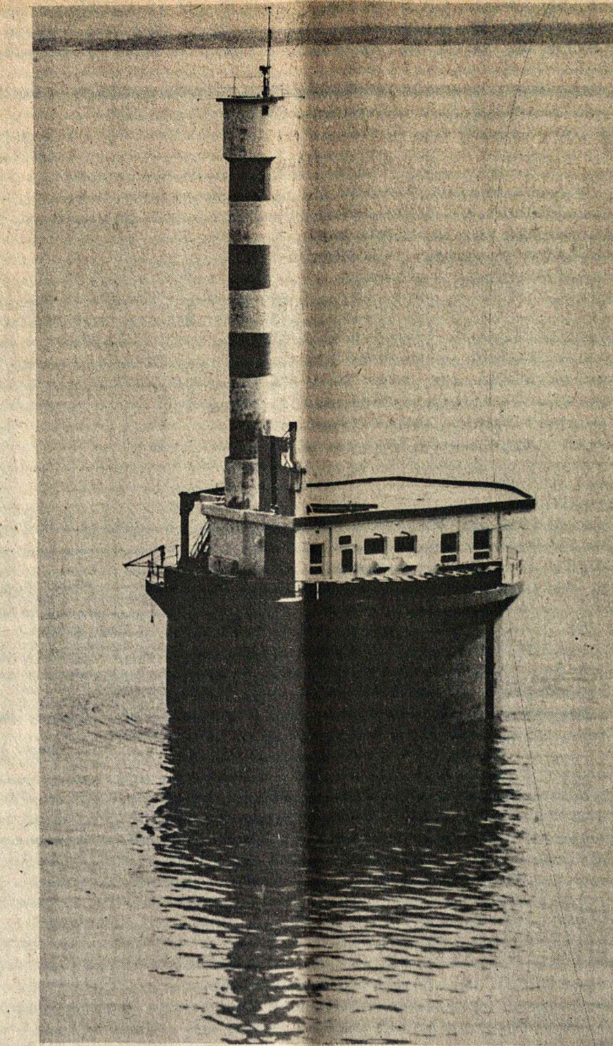
Brule Bank švyturys Lauryno upėje, 50 mylių į vakarus nuo Quebec miesto. Pastatė Department of Transport of Canada, projektavimą atliko inž. J. V. Danys. / Iš lietuvių inž. ir arch. suvažiavimo Ottawoje parodos. Nuotrauka Department of Transport/.
