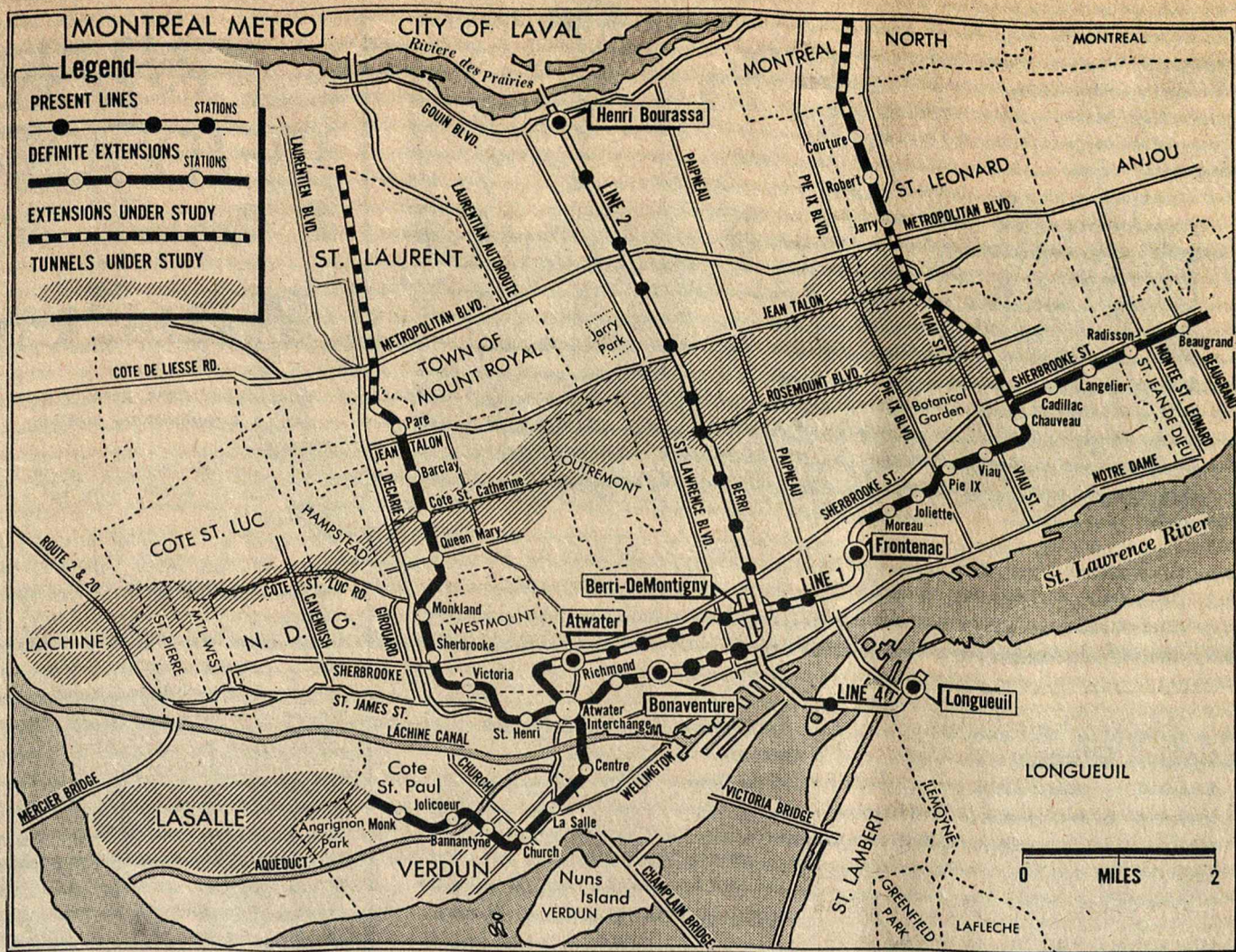
Dabartinių ir planuojamų Montrealeio metro ruožų planas
