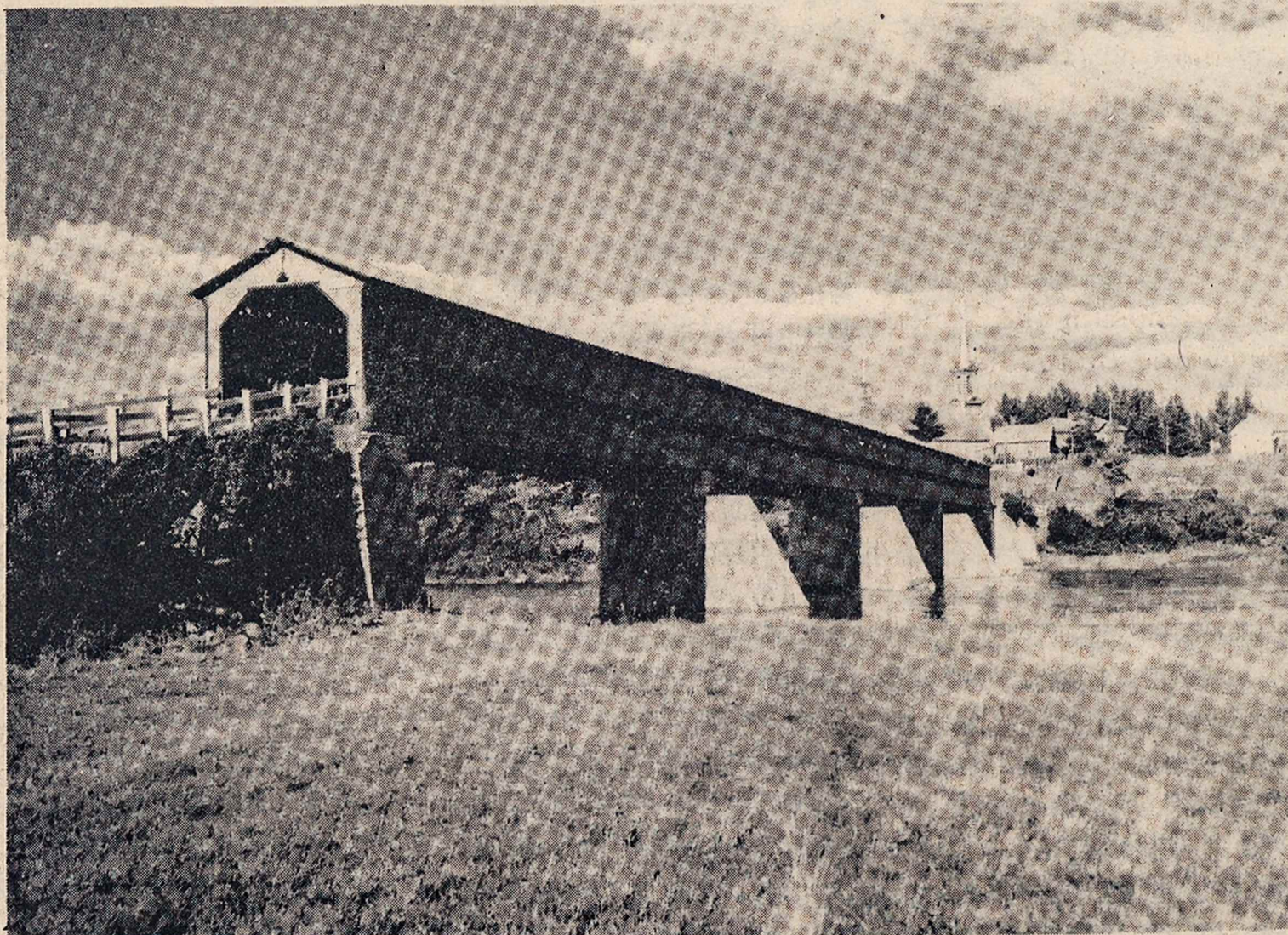
Kvebeko provincijoje vis dar yra 250 medinių dengtų tiltų — tai senosios statybos palikimas. OIP nuotraukoje matome tokį 495 pėdų ilgio tiltą Notre-Dame-la-Providence vietovėje, kertantį Chaudiere upę pietiniame Kvebeke.
