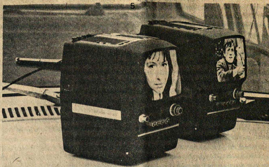
KAUNO "BANGOS" RADIO GAMYKLA SUKONSTUAVO IR SERIJOMIS GAMINA TELEVIZIJOS APARATĄ "ŠILELĮ".
