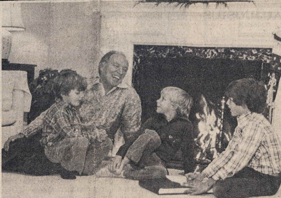
Su šia nuotrauka pasveikino "NL" ir skaitytojus Kanados Min.P-kas P.E. TRUDEAU
