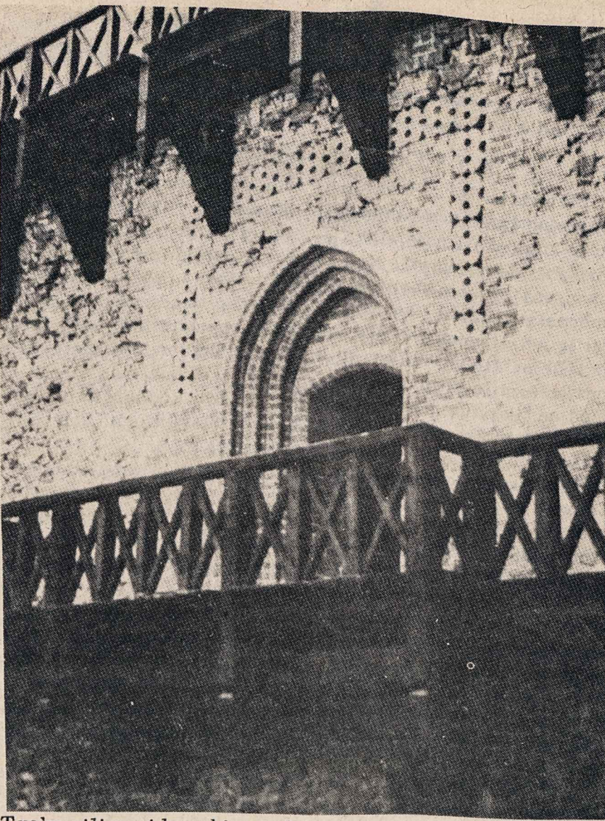
Trakų pilies vidaus kiemo dalis
