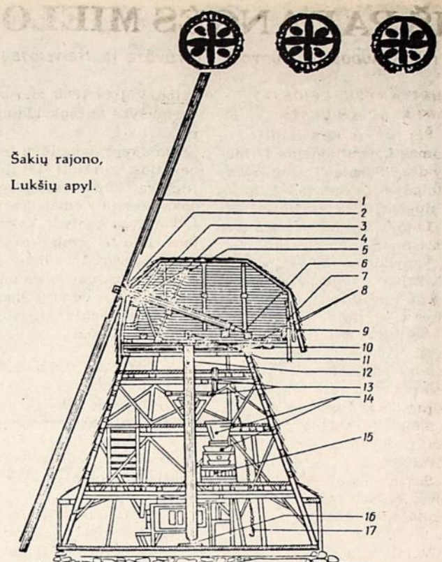
28 pav. Kepurinio malūno (Vaivadiškių) pjūvis: 1 — sparnas, 2 — sparninio veleno galva, 3 — sparninis velenas, 4 — sparninis krumpliaratis, 5 — akmeninis sparninio veleno kaklo guolis, 6 — sparninio veleno laibgalio guolis ant reguliuojamosios sijos, 7 — virvės skriemulys krumplinei gręžimo pavaraui rądomis sukti, 8 — krumpline pavara, 9 — kepurė, 10 — malūno liemens kaklas su krumpliaratėju juosta, 11 — statvolio viršutinio guolio reguliuojamoji sija, 12 — statvolis, 13 — maišų kelimo mechanizmo frukcinė pavara, 14 — piltuvė ir mechanizmas grūdams berui, 15 — girnų kubilas, 16 — statvolio apatinis reguliuojamasis guolis, 17 — maišų kelimo grandinė
