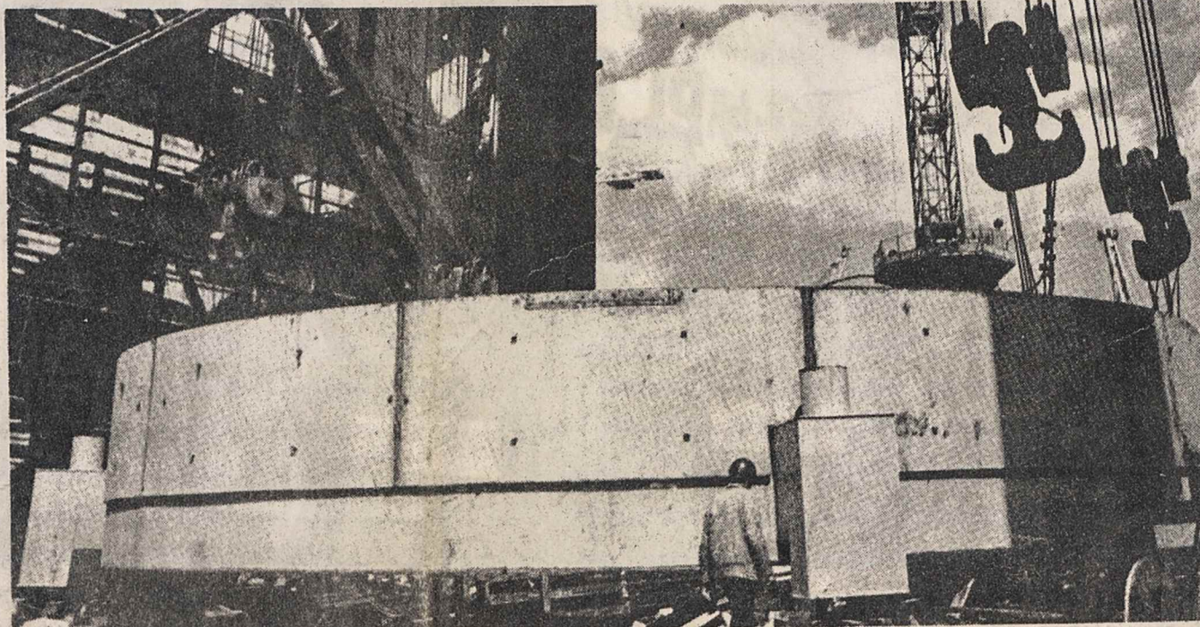
Ignalinos jėgainės reaktoriaus įmontavimo eiga.
