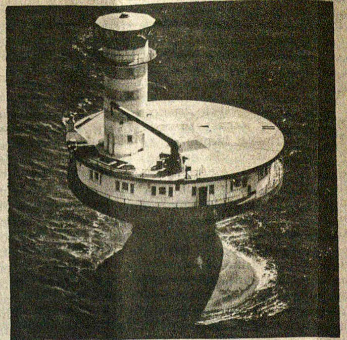
Pav. 3. Pirmasis Kanados švyturius su helikopterio platforma Prince Shoal pastatytas 1963 m.
