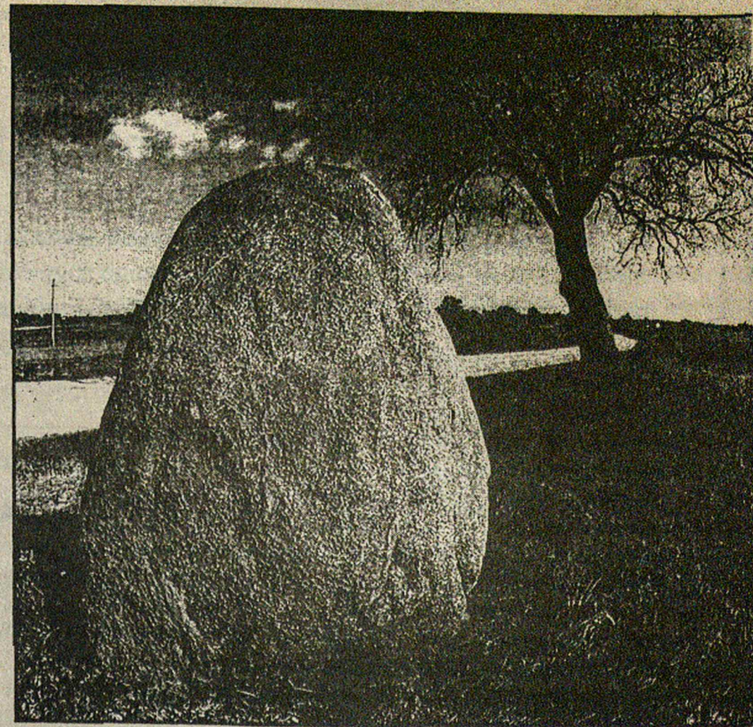
Vienas ledynų gadinės palikuonių-riedulių Žemaitijos pakeleje.
