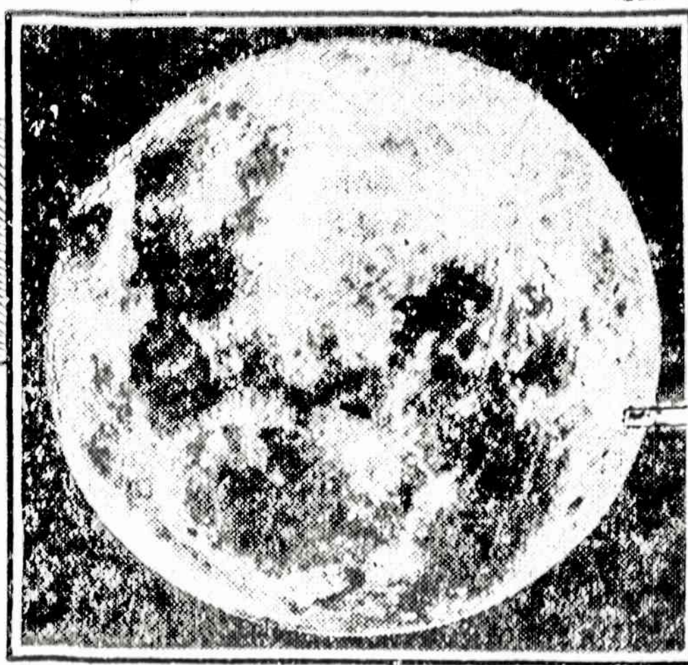
Paveikslas menulio. Virszutinis paveikslas parodo kokiū būdu atsibuna menulio užtėmimas.
