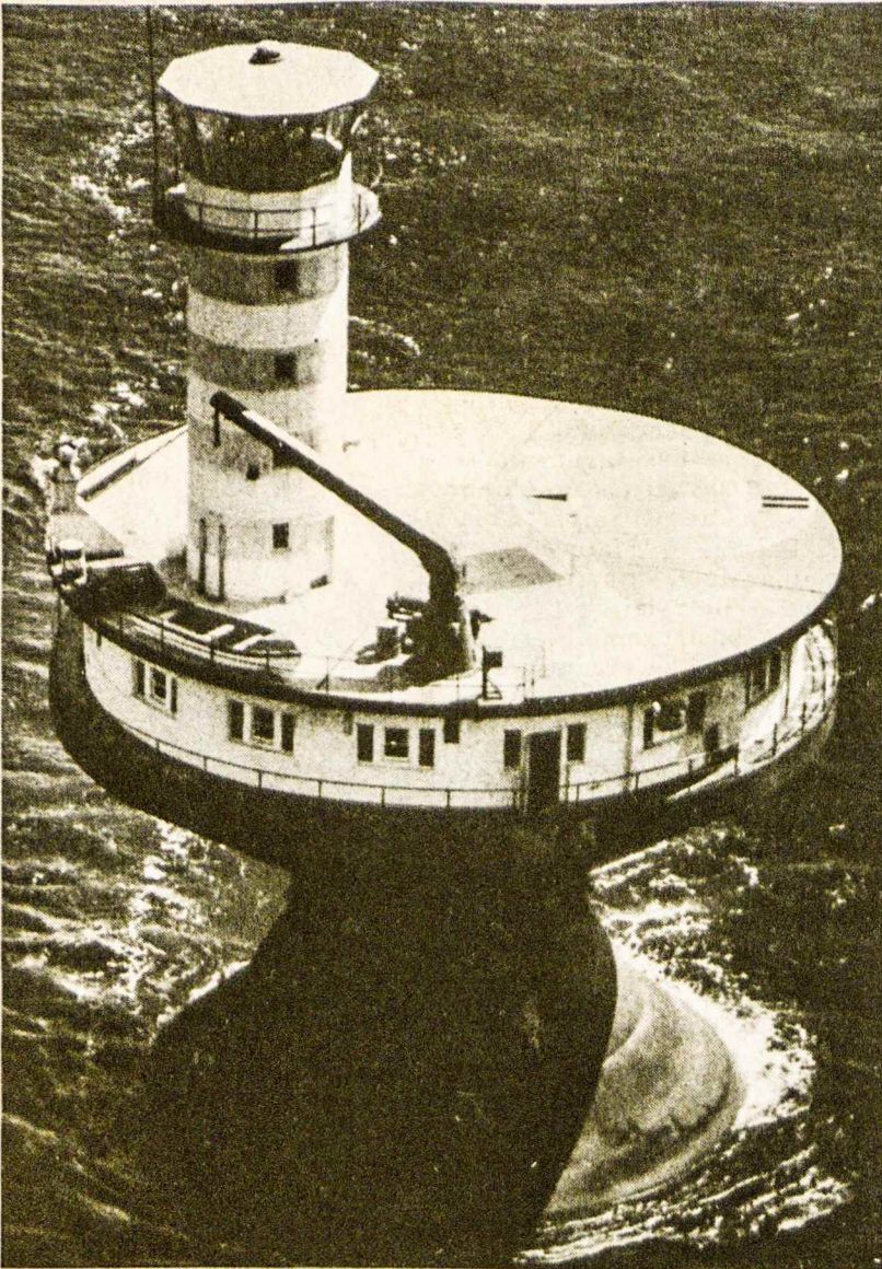
Užkrantinis švyturys Šv. Lauryno upėje Kanadoje, Haut-fond Prince (Prince Shoal), suprojektuotas ir pastatytas inž. J. V. DANIO 1964 m.
