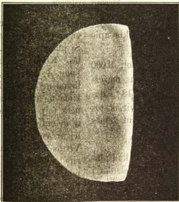
Pav. 8. Venus visada matoma puse mėnulio pavydale.
