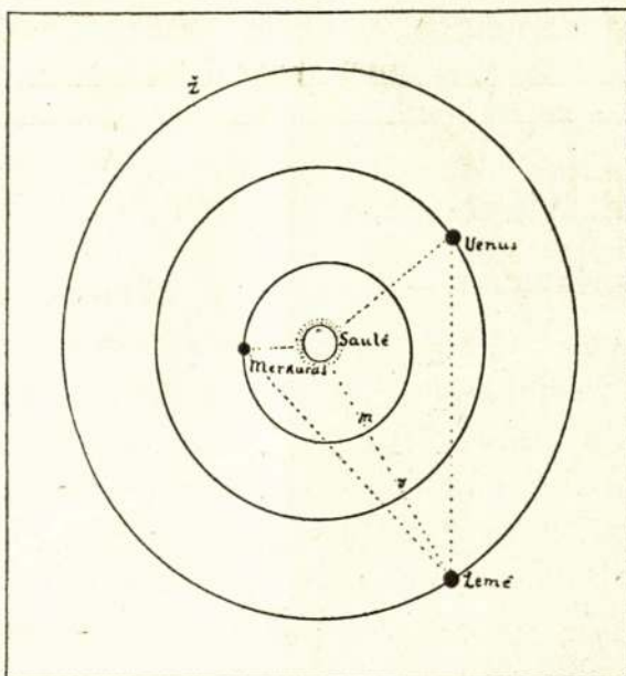
Pav. A. Merkuras, Venus ir Žemė Saulinėje Sistemoje.
