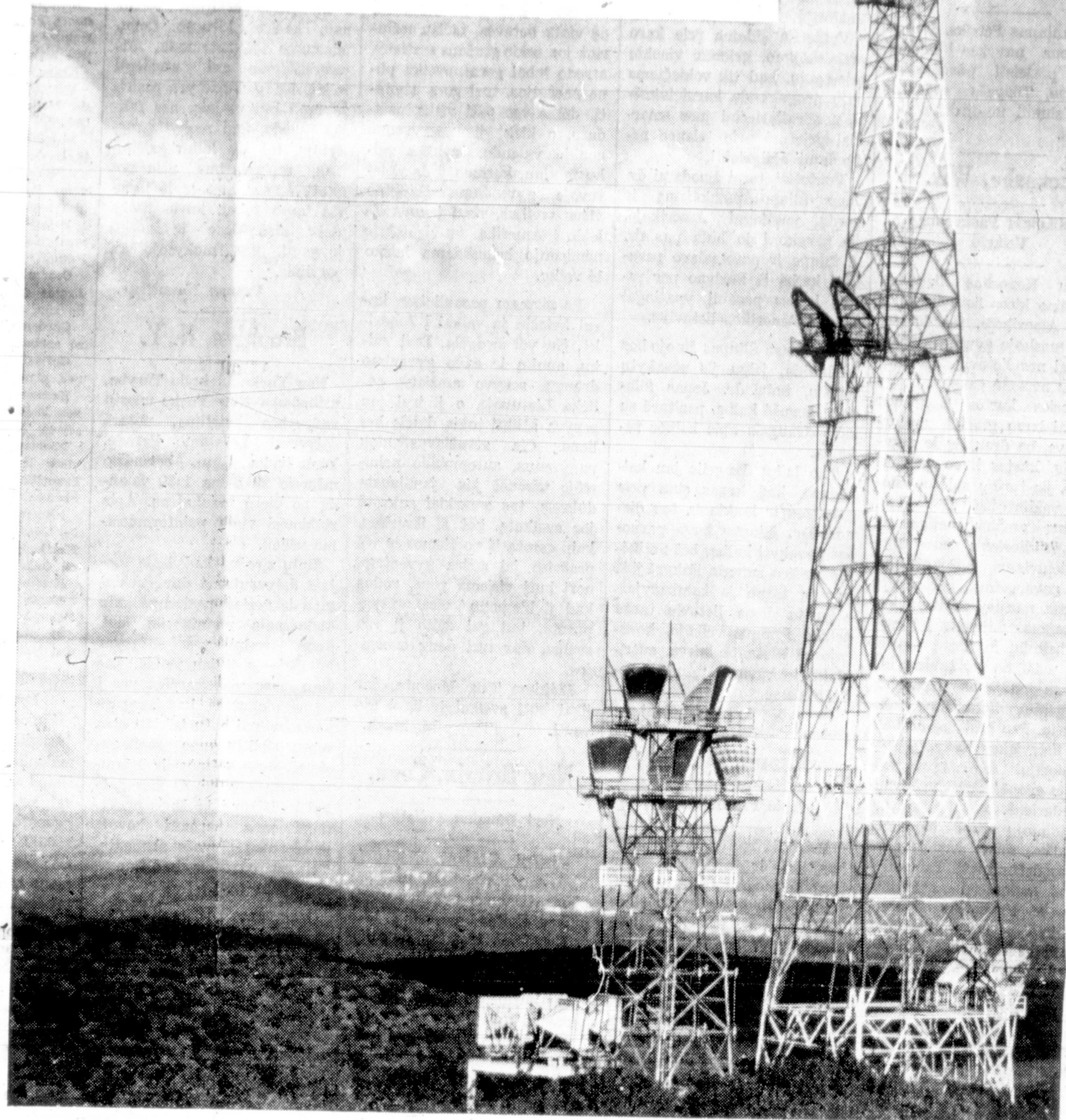
Bell Telefono trumpų bangų bokštas įrengtas New Yorko valstijoje. Jis yra Hudson upės krante ties Haverstraw.
